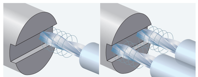
Rough Grooving
